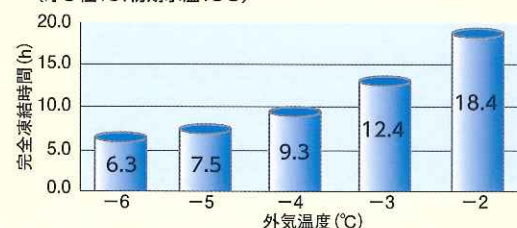
● エスロベックスCV完全凍結時間シミュレーション (呼び径13、初期水温10℃)
