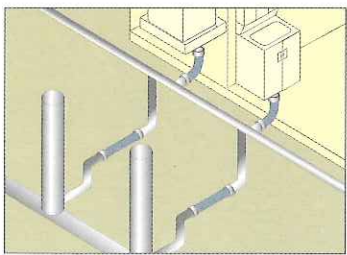
住宅地下排水(沈下・免震対策)
