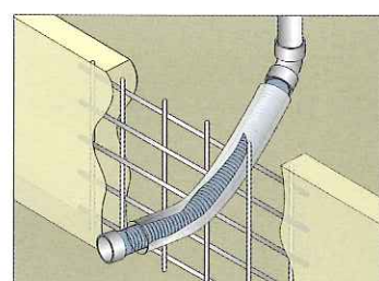
基礎貫通工法用内管
