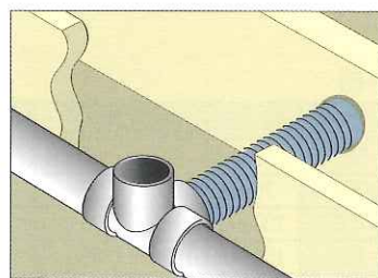
建物埋設排水配管(沈下・免震対策)
