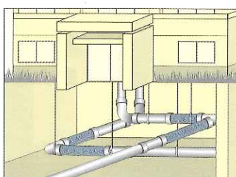
免震システム用フレキ
