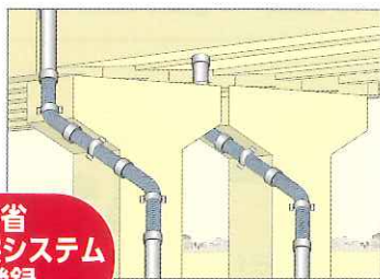
橋梁・高架排水
